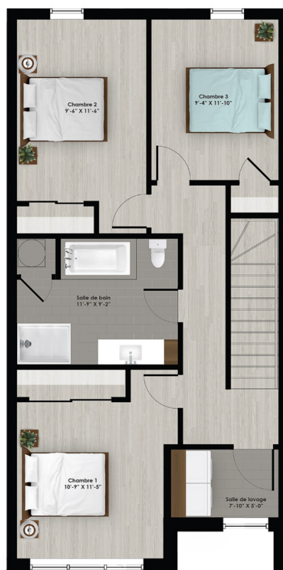
Étage
