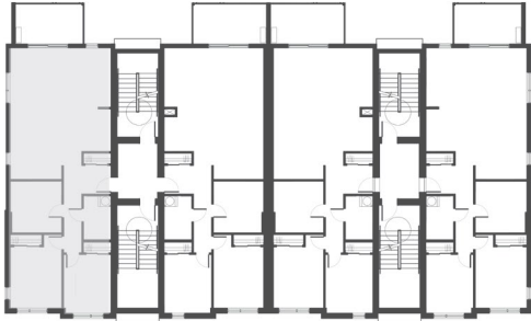
PLANCHER TYPE
